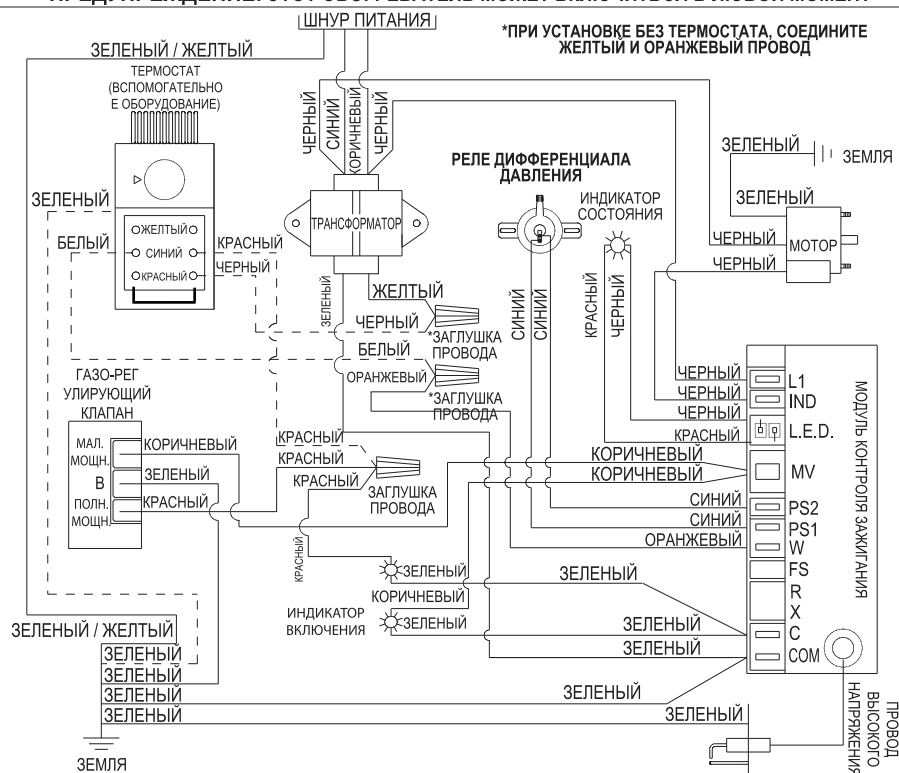
СХЕМА ЭЛЕКТРИЧЕСКИХ СОЕДИНЕНИЙ
