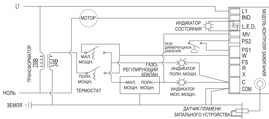
ПРИНЦИПИАЛЬНАЯ СХЕМА
