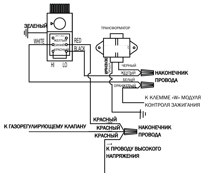
РИС. 16 2-Х СТУПЕНЧАТЫЙ ТЕРМОСТАТ
